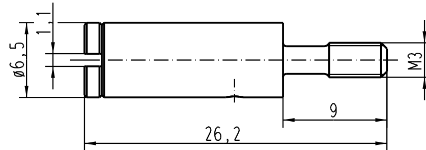
Führungsbuchse/ guide bush
