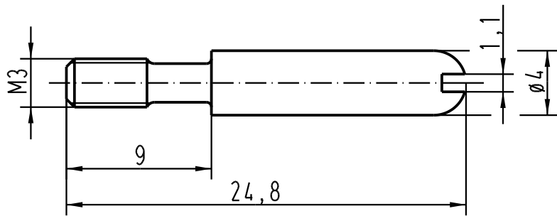
Führungsstift/ guide pin
